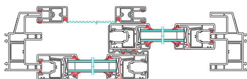
Bên trong - Inside
