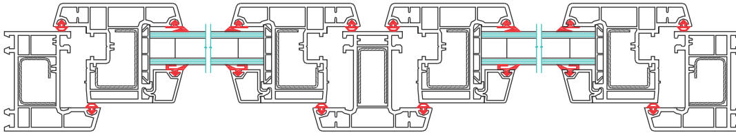
Bên trong - Inside
