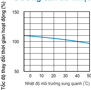
Đường cân bù nhiệt độ
