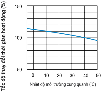
Đường cân bù nhiệt độ
