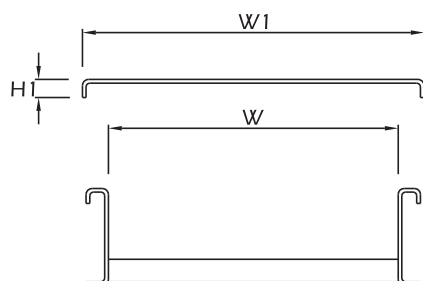
MẶT CẮT THANG CÁP VÀ NẮP ĐẨY
