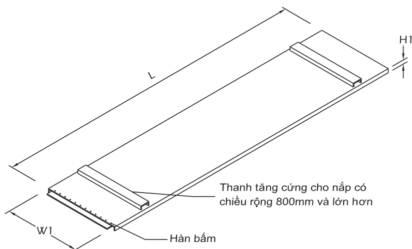
NẮP ĐẨY - VL/LG/SC
