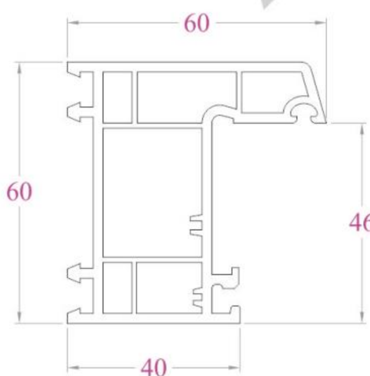
KHUÔN CỬA BR60 - 1069 g/m
