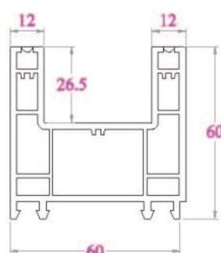
KHUÔN CỬA TRƯỢT HF62 - 1273 g/m
