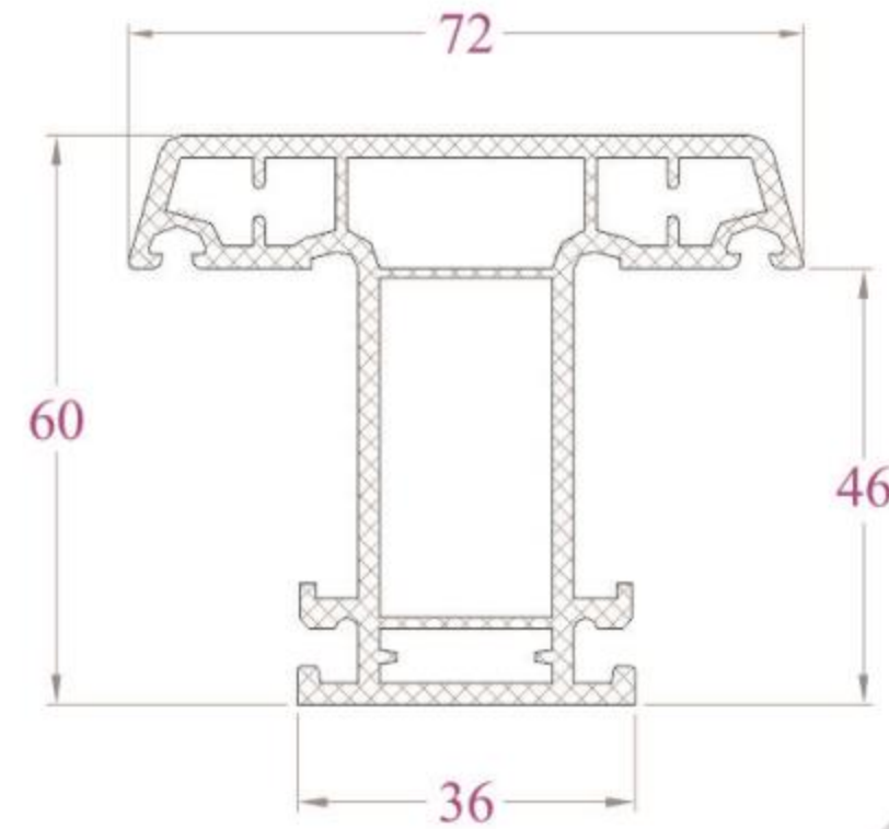
ĐỒ CỐ ĐỊNH - UP72NC 1148 g/m
