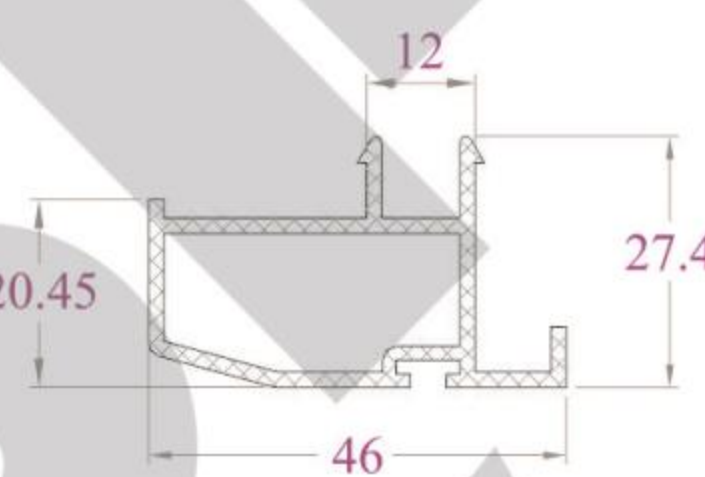
BÍT ĐÁY CỬA - HB46NC 337 g/m
