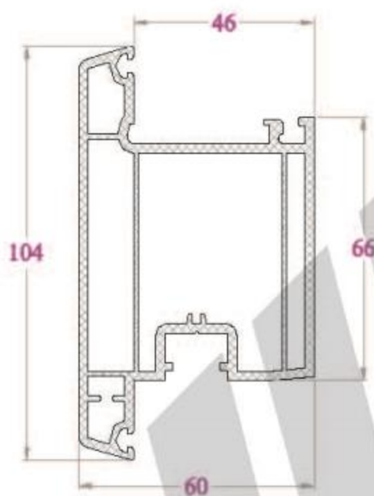
KHUNG CỬA - SF104NC 1468 g/m
