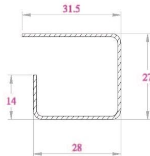
LỖI THÉP ST27x31.5 DÙNG CHO THANH BR80
