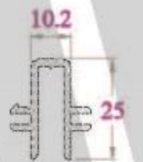
NỐI THẲNG CP6NC - 193 g/m
