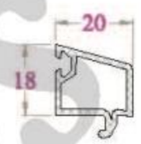
NẸP KÍNH - GB19NC 196 g/m (Kính hộp 16, Pano)
