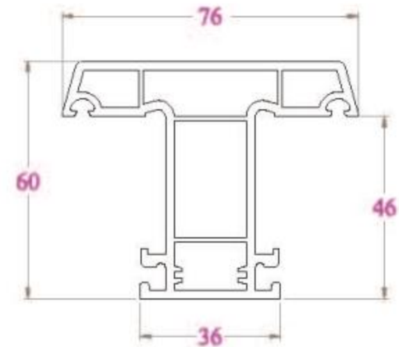
ĐỒ CỐ ĐỊNH SE76N - 1119 g/m
