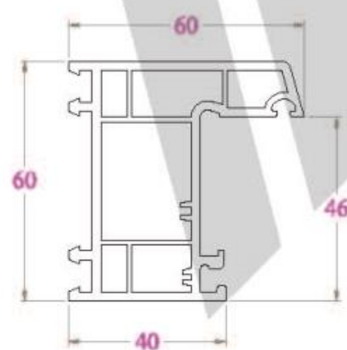
KHUÔN CỬA - BR60 1069 g/m
