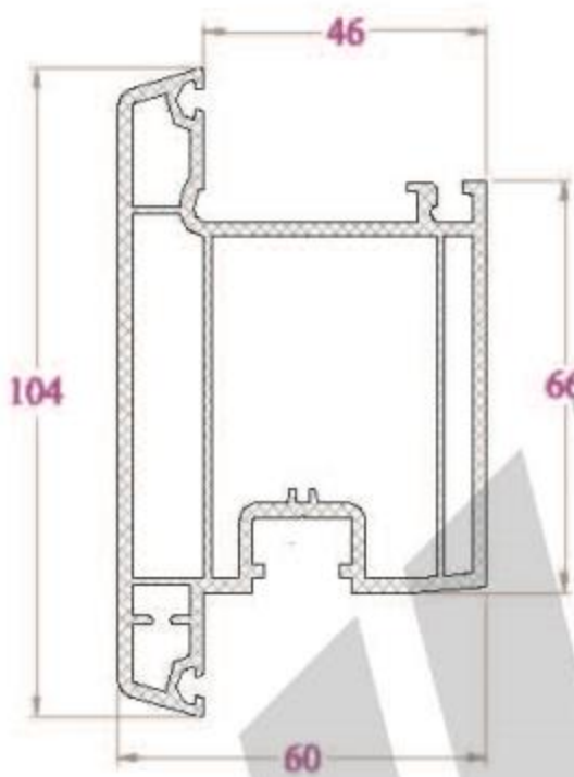
KHUNG CỬA - SF104NC 1468 g/m
