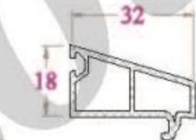
NẸP KÍNH - GB31NC 272 g/m (Kính đơn 8)
