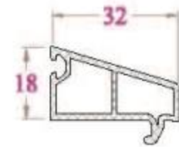
NẸP KÍNH GB31NC 272 g/m (Kính đơn 8)
