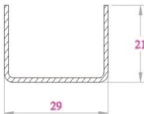
LỖI THÉP ST29x21 DÙNG CHO THANH HF62 VÀ HF95N
