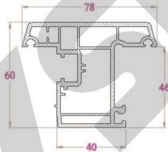
KHUNG CỬA - SF78NC 1178 g/m
