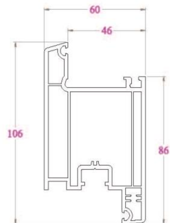
KHUNG CỬA FR106 - 1514 g/m
