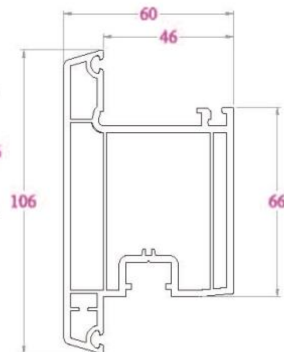
KHUÔN CỬA SF106 - 1540 g/m
