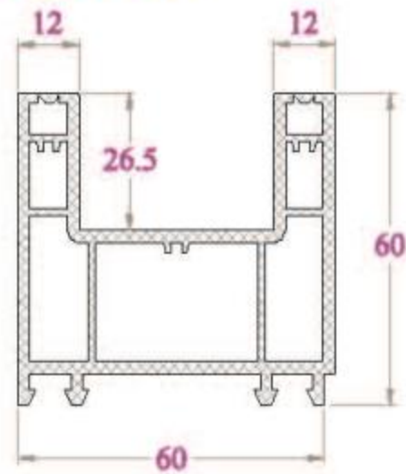
KHUÔN CỬA TRƯỢT - HF60NC 1250 g/m
