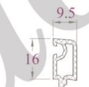
NỆP KÍNH - GB10NC 137 g/m (Kính hộp 20)
