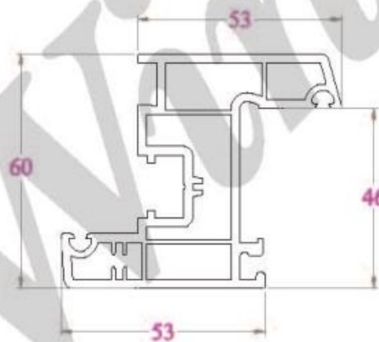
KHUÔN CỬA FR73N - 1140 g/m
