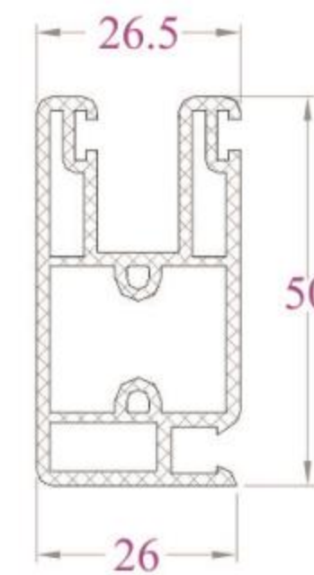
KHUNG LẮP LƯỚI MF50NC - 595 g/m
