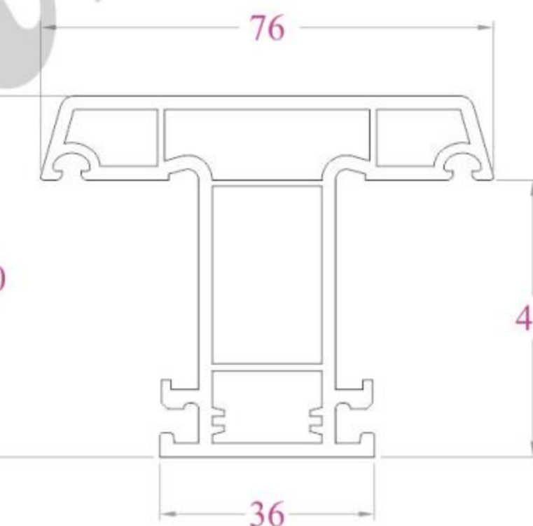
ĐỒ CỐ ĐỊNH SE76N - 1119 g/m
