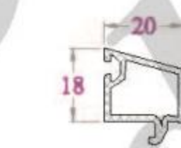
NẸP KÍNH - GB19NC 196 g/m (Kính hộp 16, Pano)
