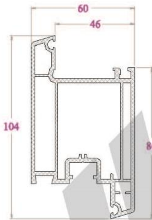
KHUÔN CỬA - FR104NC 1545 g/m
