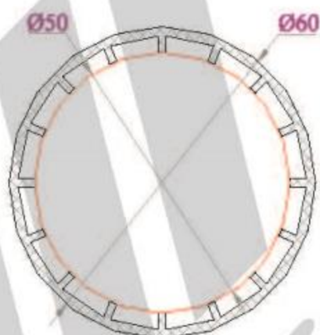
TRỤ CHUYỂN HƯỚNG 90° ÷ 180° TP60NC - 805 g/m
