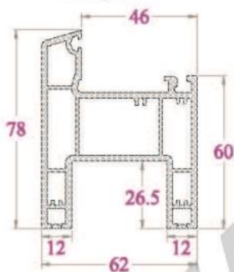
KHUÔN CỬA TRƯỢT LIÊN VÁCH YT62 - 1404 g/m
