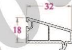
NẸP KÍNH GB31NC 272 g/m (Kính đơn 8)
