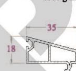
NẸP KÍNH - GB34NC 277 g/m (Kính đơn 5)
