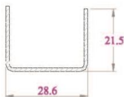
LỖI THÉP ST30x21.5 DÙNG CHO THANH HF60NC VÀ HF95NC
