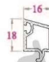
NẾP KÍNH - GB15NC 163 g/m (Kính hộp 20)
