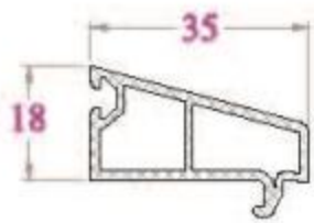
NẸP KÍNH - GB34NC 277 g/m (Kính đơn 5)
