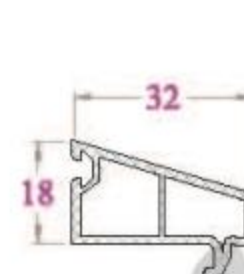
NẸP KÍNH GB31NC 272 g/m (Kính đơn 8)
