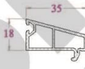
NẸP KÍNH - GB34NC 277 g/m (Kính đơn 5)
