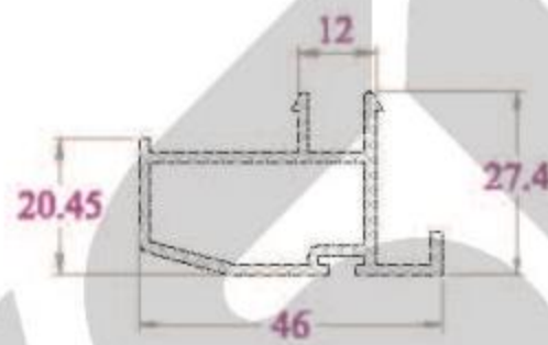
BỊT ĐÁY CỬA - HB46NC 337 g/m
