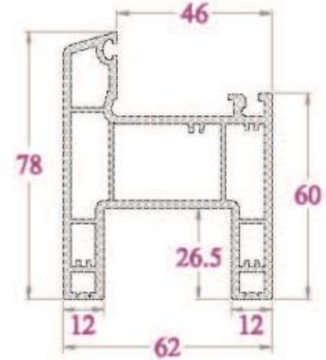
KHUÔN CỬA TRƯỢT LIÊN VÁCH YT62 - 1404 g/m
