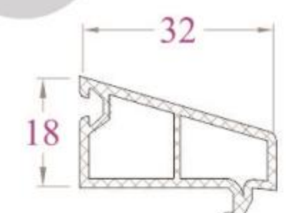
NẸP KÍNH GB31NC 272 g/m (Kính đơn 8)
