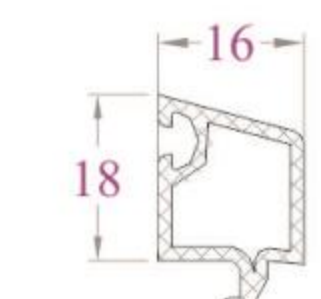
NẸP KÍNH - GB15NC 163 g/m (Kính hộp 20)
