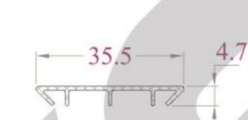
ĐỆM KÍNH - FL36NC 85 g/m
