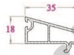
NẸP KÍNH - GB34NC 277 g/m (Kính đơn 5)
