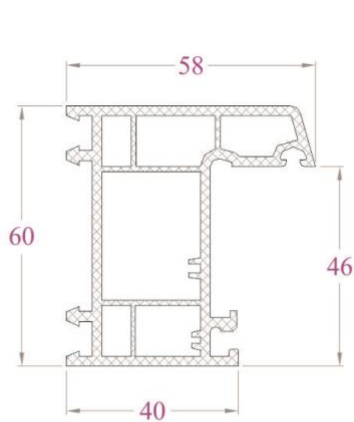
KHUÔN CỬA - BR58NC 1030 g/m
