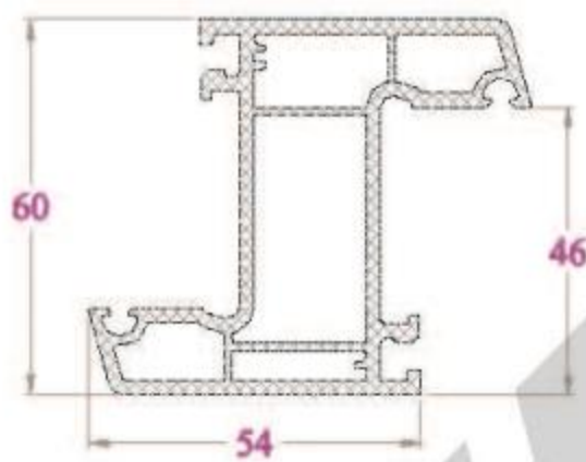
ĐỒ CỐ ĐỊNH - KP72NC 1059 g/m
