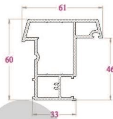
ĐỒ GIẢ GIỮA - ST61NC 912 g/m
