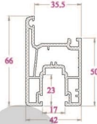
KHUNG CỬA - SF66NC 1000 g/m
