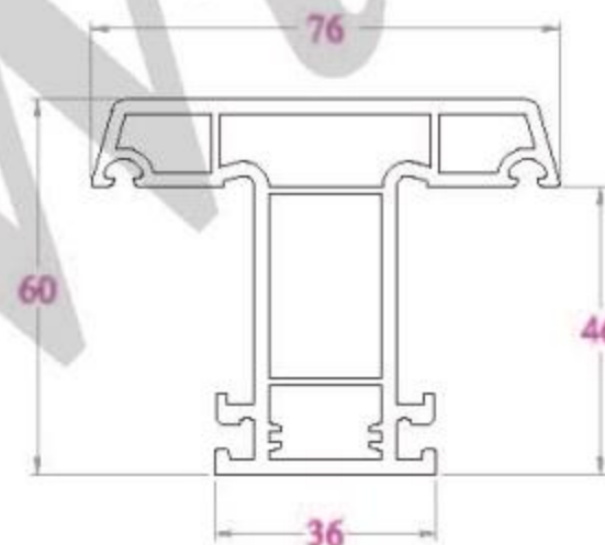
ĐỒ CỐ ĐỊNH SE76N - 1119 g/m
