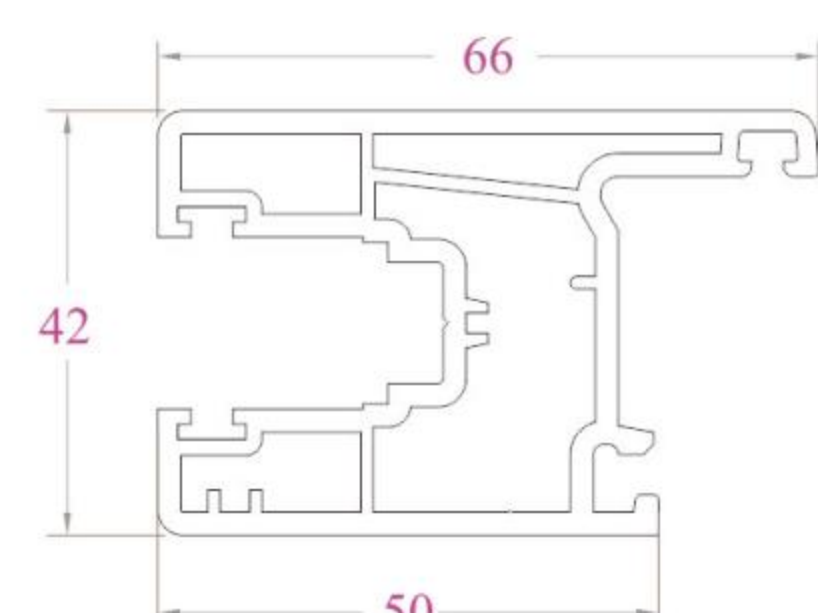
KHUÔN CỬA TRƯỢT SF66 - 1003 g/m
