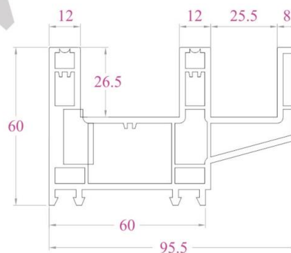
KHUÔN CỬA TRƯỢT HF95 1685 g/m
