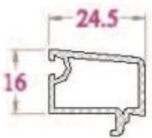
NỆP KÍNH - GB25NC 218 g/m (Kính đơn 5)
