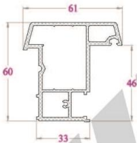
ĐỒ GIẢ GIỮA(2a) - ST61NC 912 g/m
