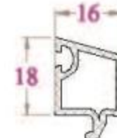
NẸP KÍNH - GB15NC 163 g/m (Kính hộp 20)
