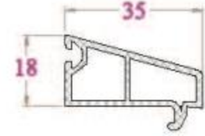
NẾP KÍNH - GB34NC 277 g/m (Kính đơn 5)
