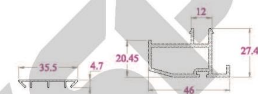
ĐỆM KÍNH - FL36NC 85 g/m
