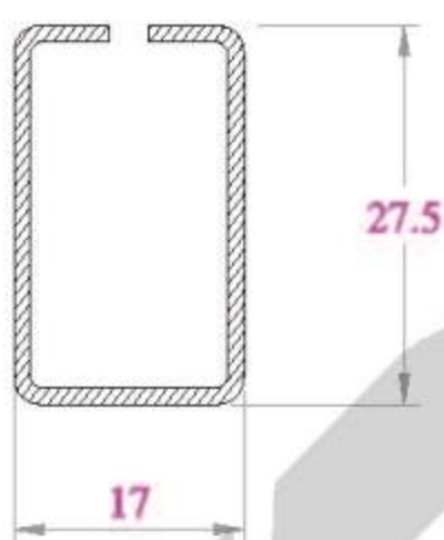
LỖI THÉP ST27.5x17 DÙNG CHO THANH SE76N
