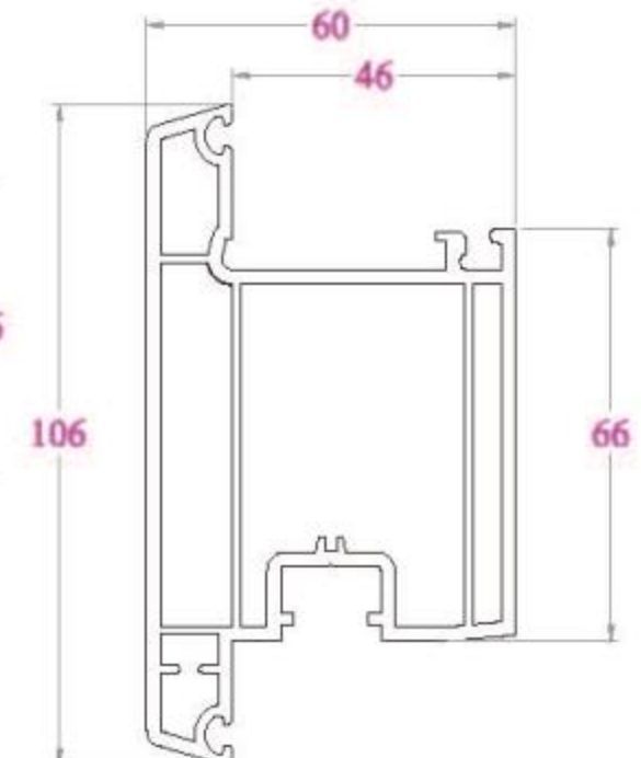
KHUNG CỬA SF106 - 1540 g/m
