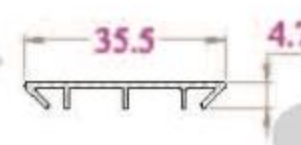
ĐỆM KÍNH - FL36NC 85 g/m
