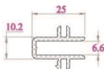
NỐI THẲNG CP6NC - 193 g/m
