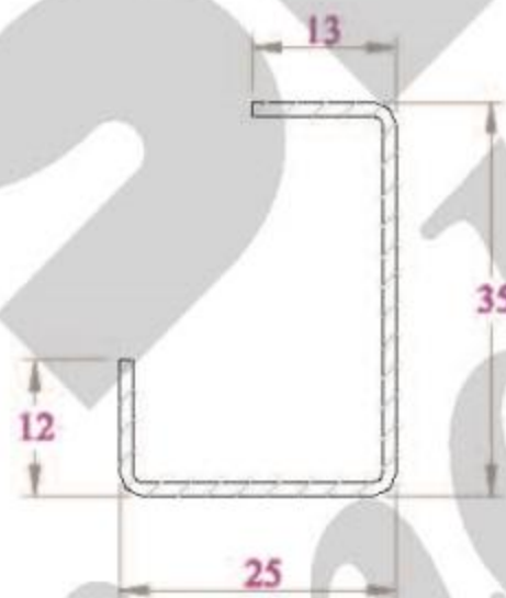
LỖ THÉP STC35x27.5 DÙNG CHO THANH SF78NC
