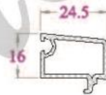
NẸP KÍNH - GB25NC 218 g/m (Kính đơn 5)
