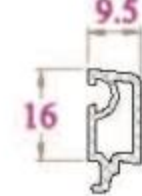
NẸP KÍNH - GB10NC 137 g/m (Kính hộp 20)
