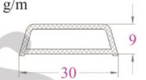
NẠP TRANG TRÍ ZS30 - 210 g/m
