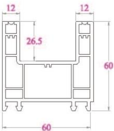
KHUÔN CỬA TRƯỢT HF62 - 1273 g/m
