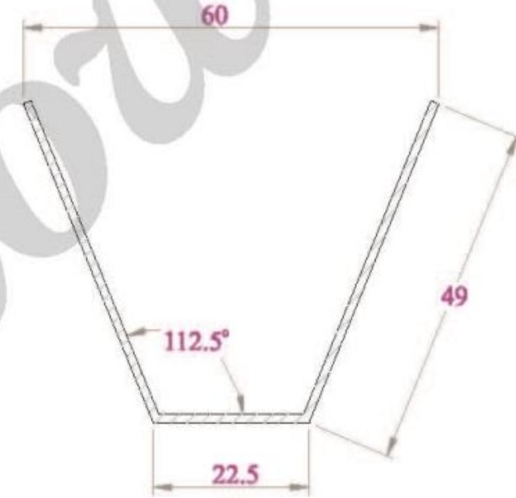
LỖI THÉP ST60x49 DÙNG CHO THANH TC60NC
