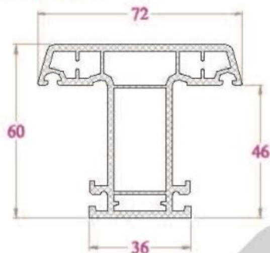
ĐỒ CỐ ĐỊNH - UP72NC 1148 g/m
