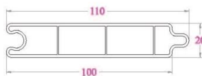
PANO CỬA - PP100N 613 g/m
