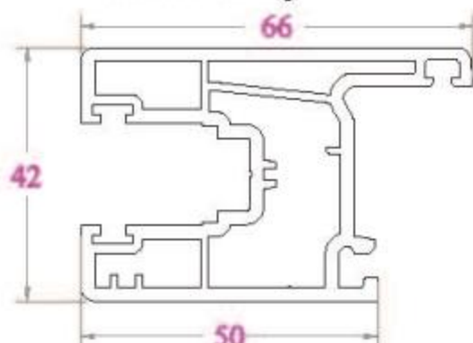
KHUÔN CỬA TRƯỢT SF66 - 1003 g/m
