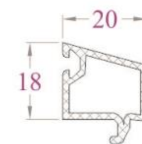
NỆP KÍNH - GB19NC 196 g/m (Kính hộp 16, Pano)
