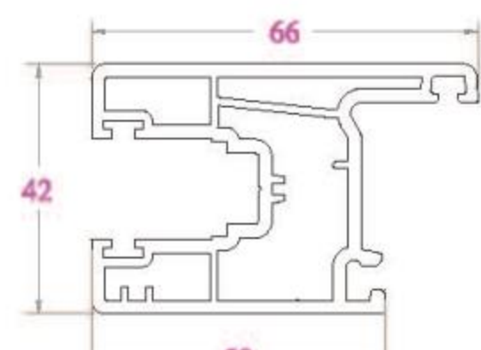
KHUÔN CỬA TRƯỢT SF66 - 1003 g/m
