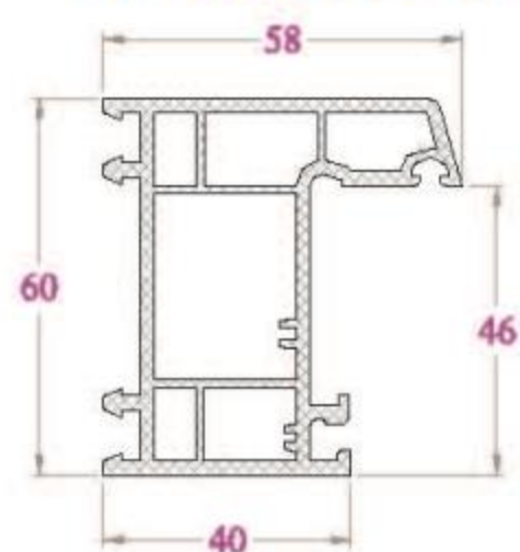
KHUÔN CỬA - BR58NC 1030 g/m
