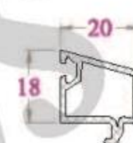
NẸP KÍNH - GB19NC 196 g/m (Kính hộp 16, Pano)
