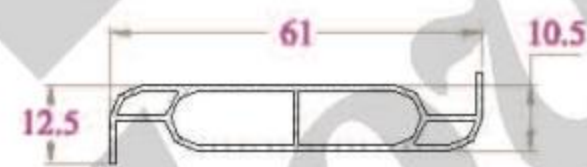
LÁ CHÓP - LP61NC 267 g/m
