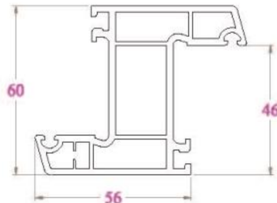
ĐỒ CỐ ĐỊNH - PZ76N 1091 g/m
