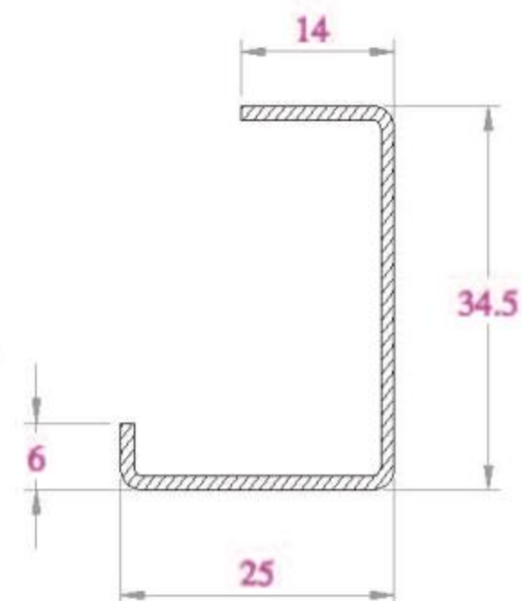
LỖI THÉP ST34.5x25 DÙNG CHO THANH SF78C
