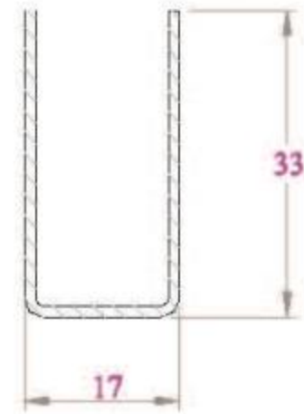
LỖ THÉP ST35x17 DÙNG CHO THANH UP72NC VÀ KP72NC
