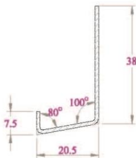
LỖ THÉP STC41x20.5 DÙNG CHO THANH FR71NC
