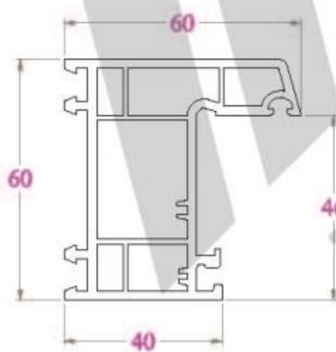
KHUÔN CỬA BR60 - 1069 g/m
