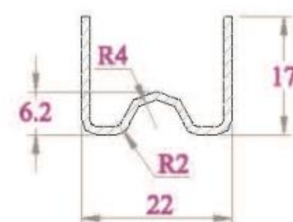
LỖI THÉP ST22x17 DÙNG CHO THANH MF50NC
