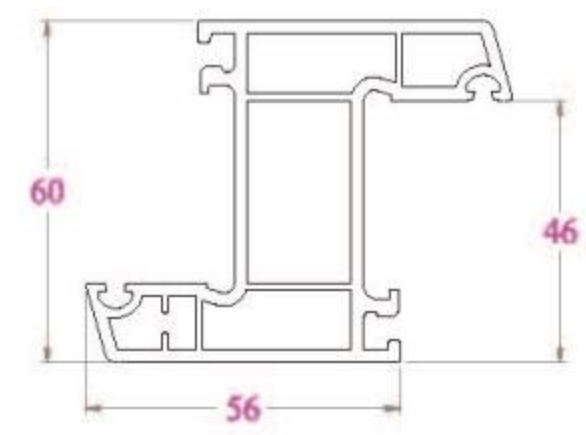
ĐỒ CỐ ĐỊNH PZ76N - 1091 g/m
