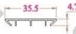
ĐỆM KÍNH - FL36NC 85 g/m
