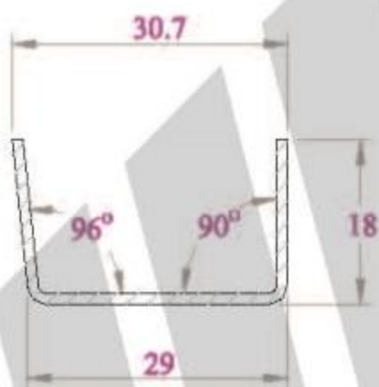
LỖ THÉP ST30x18 DÙNG CHO THANH SF66NC
