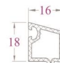
NỆP KÍNH - GB15NC 163 g/m (Kính hộp 20)
