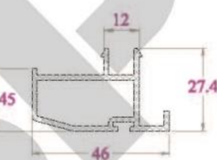
BỊT ĐÁY CỬA - HB46NC 337 g/m
