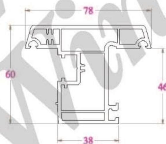
KHUNG CỬA - SF78C 1009 g/m
