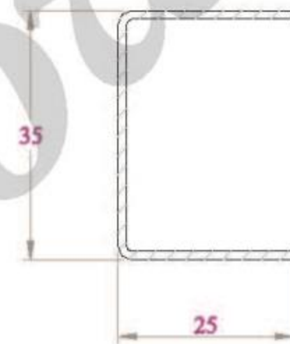
LỖ THÉP STC35x25 DÙNG CHO THANH ST61NC
