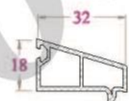
NẸP KÍNH GB31NC 272 g/m (Kính đơn 8)
