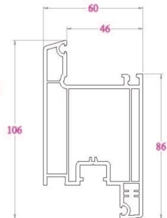
KHUÔN CỬA - FR106 1514 g/m
