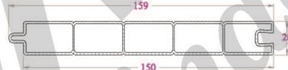
PANO CỬA - PP150NC 900 g/m
