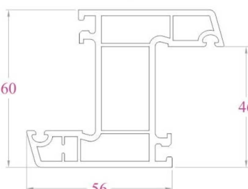
ĐỒ CỐ ĐỊNH PZ76N - 1091 g/m
