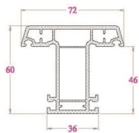
ĐỒ CỐ ĐỊNH - UP72NC 1148 g/m
