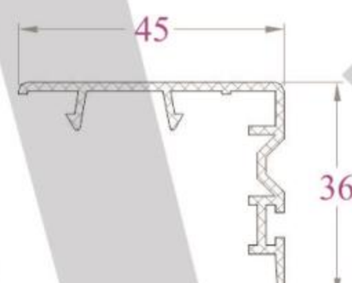
BÍT ĐẦU KHUNG - IL36NC 233 g/m
