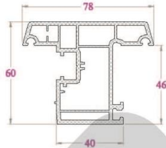
KHUNG CỬA - SF78NC 1178 g/m
