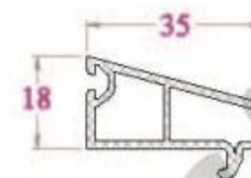
NẸP KÍNH - GB34NC 277 g/m (Kính đơn 5)
