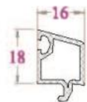
NẸP KÍNH - GB15NC 163 g/m (Kính hộp 20)
