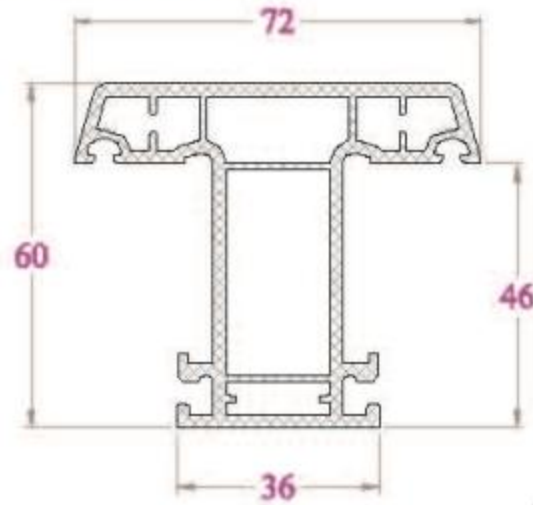
ĐỒ CỐ ĐỊNH - UP72NC 1148 g/m
