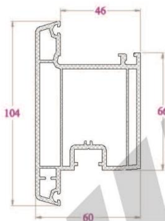
KHUÔN CỬA - SF104NC 1468 g/m
