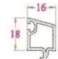
NẸP KÍNH - GB15NC 163 g/m (Kính hộp 20)
