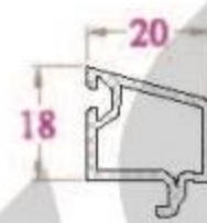
NẸP KÍNH - GB19NC 196 g/m (Kính hộp 16, Pano)
