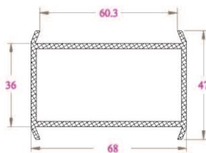
NỐI THẲNG CP47NC - 809 g/m
