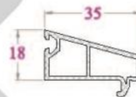
NẸP KÍNH - GB34NC 277 g/m (Kính đơn 5)
