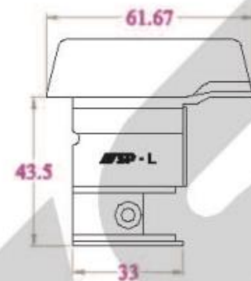
ĐẦU BÍT TRÁI - DB61NC/T
