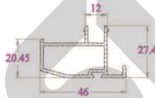
BẬT ĐÁY CỬA - HB46NC 337 g/m
