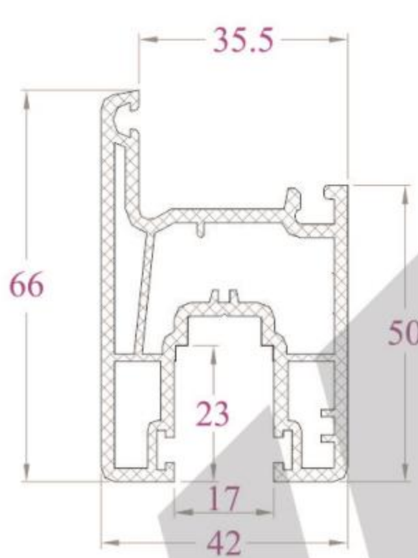
KHUNG CỬA - SF66NC 1000 g/m
