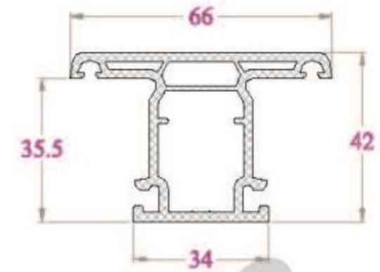
ĐÓ GIỮA SP66NC - 837 g/m
