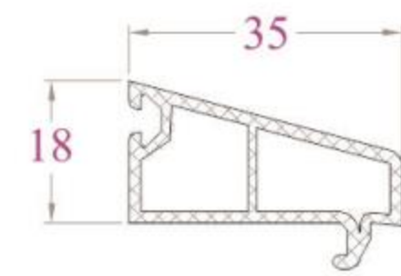
NỆP KÍNH - GB34NC 277 g/m (Kính đơn 5)
