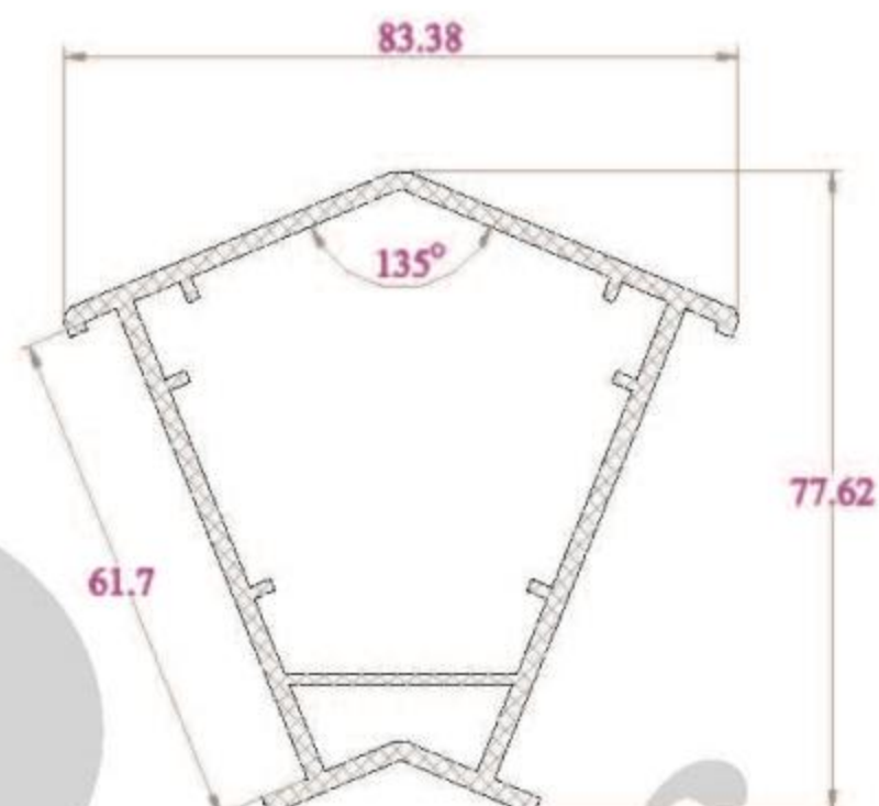
TRỤ CHUYỂN HƯỚNG 135° TC60NC - 1041 g/m
