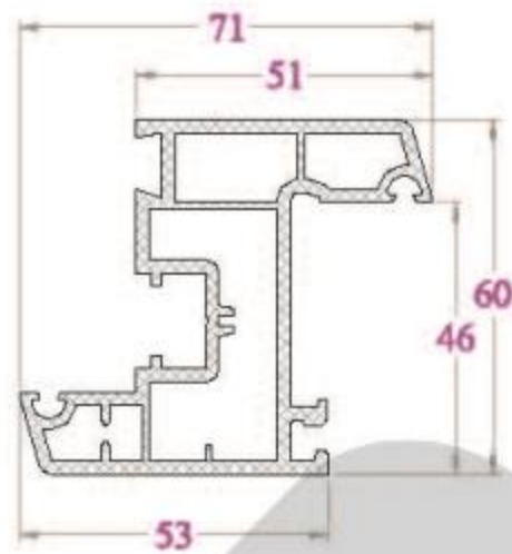
KHUÔN CỬA - FR71NC 1102 g/m
