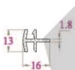
NỐI THẲNG CP2NC - 103 g/m
