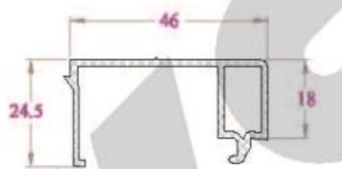
NẸP ĐỨNG LẮP CHÓP - RP45NC 312 g/m
