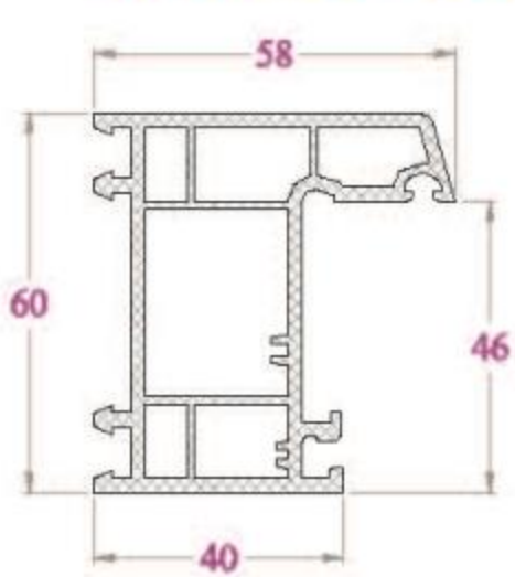
KHUÔN CỬA - BR58NC 1030 g/m
