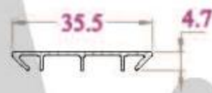
ĐỆM KÍNH - FL36NC 85 g/m
