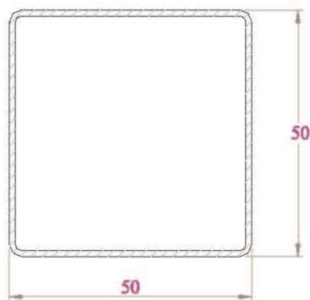
LỖI THÉP ST50x50 DÙNG CHO THANH CP90NC
