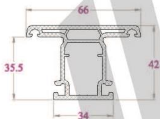
ĐỒ GIỮA SP66NC - 837 g/m
