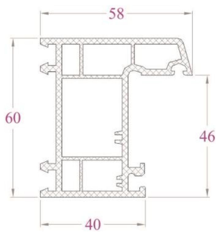
KHUÔN CỬA - BR58NC 1030 g/m
