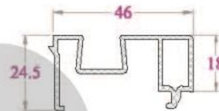
NẸP NGANG LẮP CHÓP - RP18NC 398 g/m
