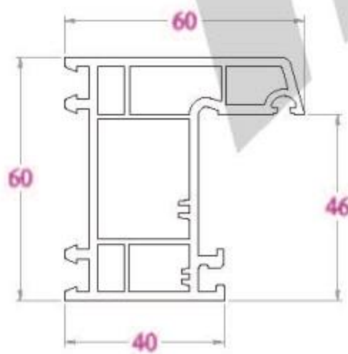
KHUÔN CỬA BR60 - 1069 g/m
