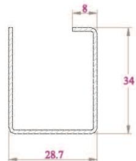
LỖ THÉP ST28x34 DÙNG CHO THANH SF92NC
