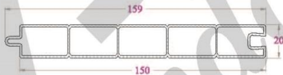
PANO CỬA - PP150NC 900 g/m
