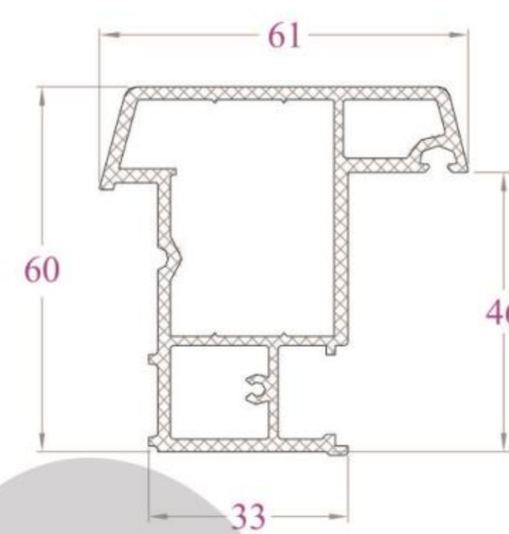
ĐỒ GIẢ GIỮA - ST61NC 912 g/m
