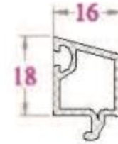
NẸP KÍNH - GB15NC 163 g/m (Kính hộp 20)
