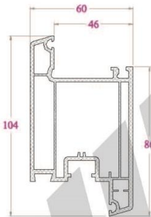
KHUNG CỬA - FR104NC 1545 g/m
