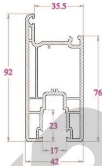
KHUNG CỬA SF92NC - 1246 g/m
