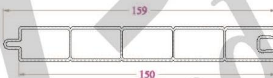
PANO CỬA - PP150NC 900 g/m
