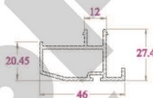
BÍT ĐÁY CỬA - HB46NC 337 g/m
