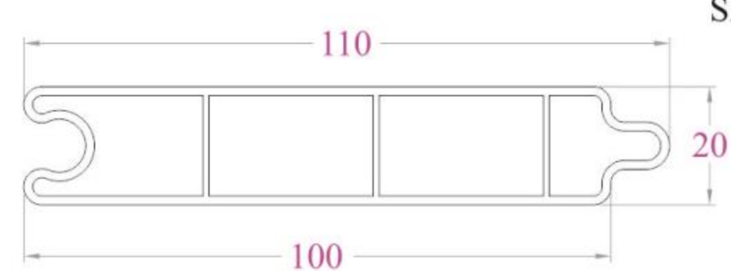
PANO CỬA - PP100N 613 g/m
