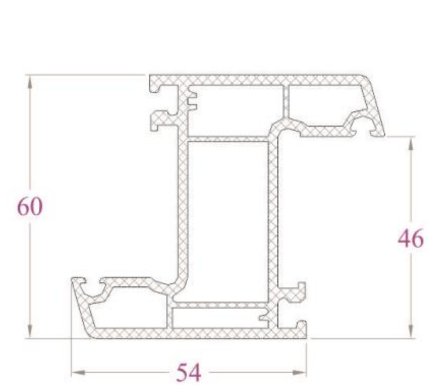
ĐỒ CỐ ĐỊNH - KP72NC 1059 g/m
