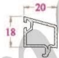
NẸP KÍNH - GB19NC 196 g/m (Kính hộp 16, Pano)
