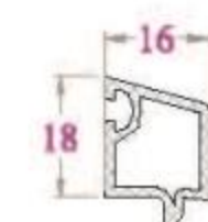
NẸP KÍNH - GB15NC 163 g/m (Kính hộp 20)
