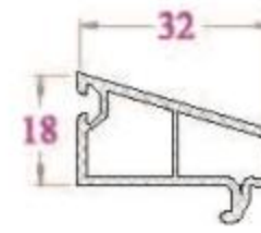
NẸP KÍNH GB31NC 272 g/m (Kính đơn 8)
