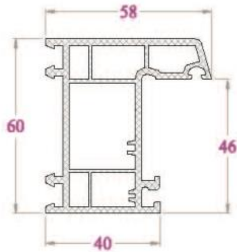
KHUÔN CỬA - BR58NC 1030 g/m
