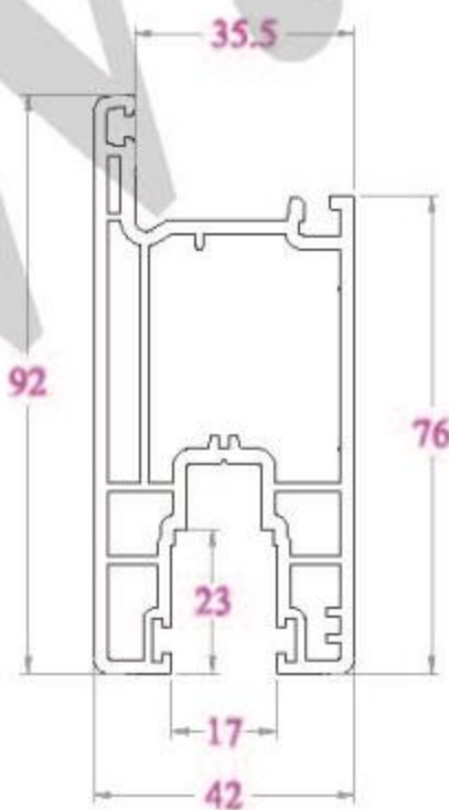
KHUNG CỬA SF92N 1254 g/m
