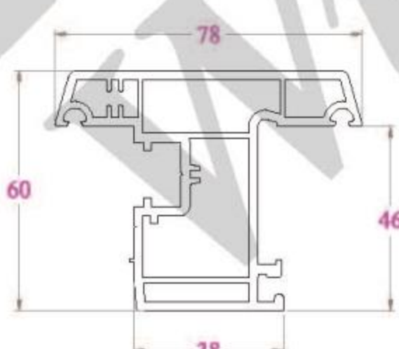
KHUNG CỬA SF78C - 1009 g/m
