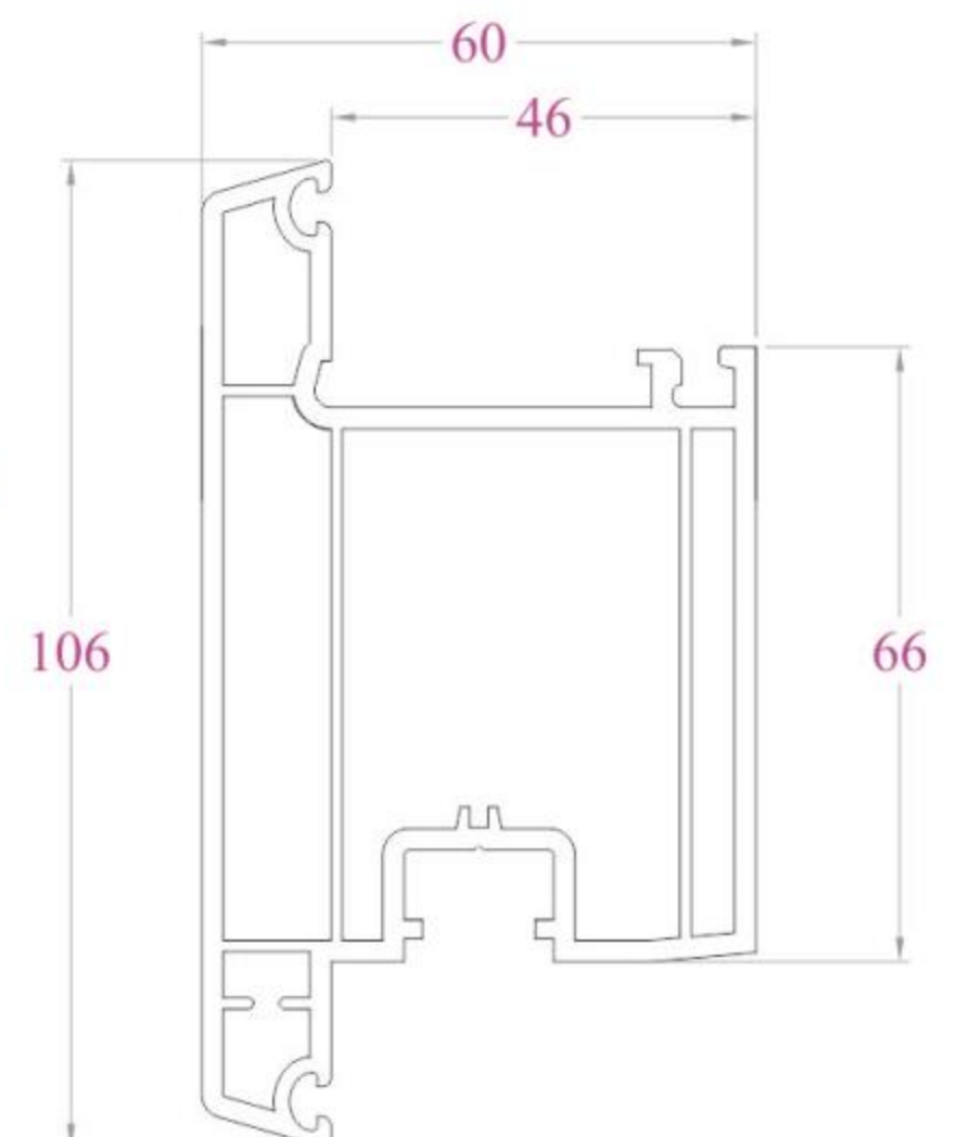
KHUÔN CỬA SF106 - 1540 g/m
