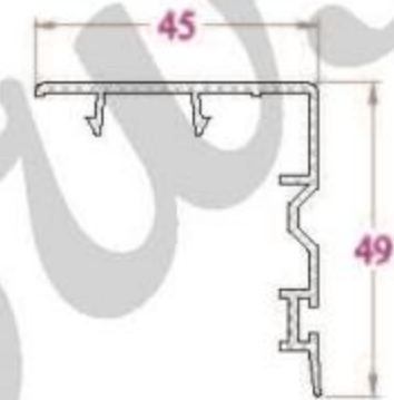
BỊT ĐẦU KHUNG IL49NC - 281 g/m
