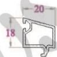
NẸP KÍNH - GB19NC 196 g/m (Kính hộp 16, Pano)
