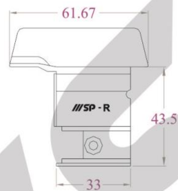
ĐẦU BÍT PHẢI DB61NC/P
