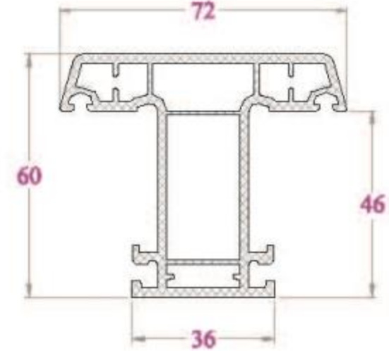
ĐỒ CỐ ĐỊNH - UP72NC 1148 g/m
