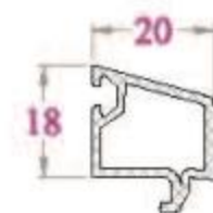
NẾP KÍNH - GB19NC 196 g/m (Kính hộp 16, Pano)
