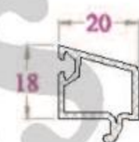
NẸP KÍNH - GB19NC 196 g/m (Kính hộp 16, Pano)
