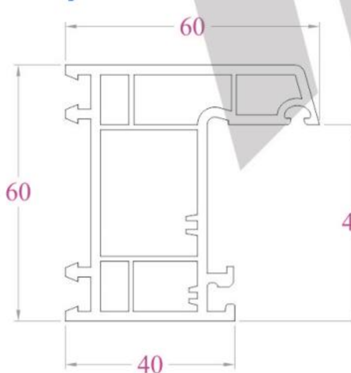
KHUÔN CỬA BR60 - 1069 g/m
