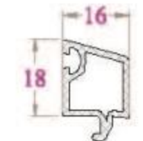
NẸP KÍNH - GB15NC 163 g/m (Kính hộp 20)
