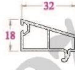
NẸP KÍNH GB31NC 272 g/m (Kính đơn 8)
