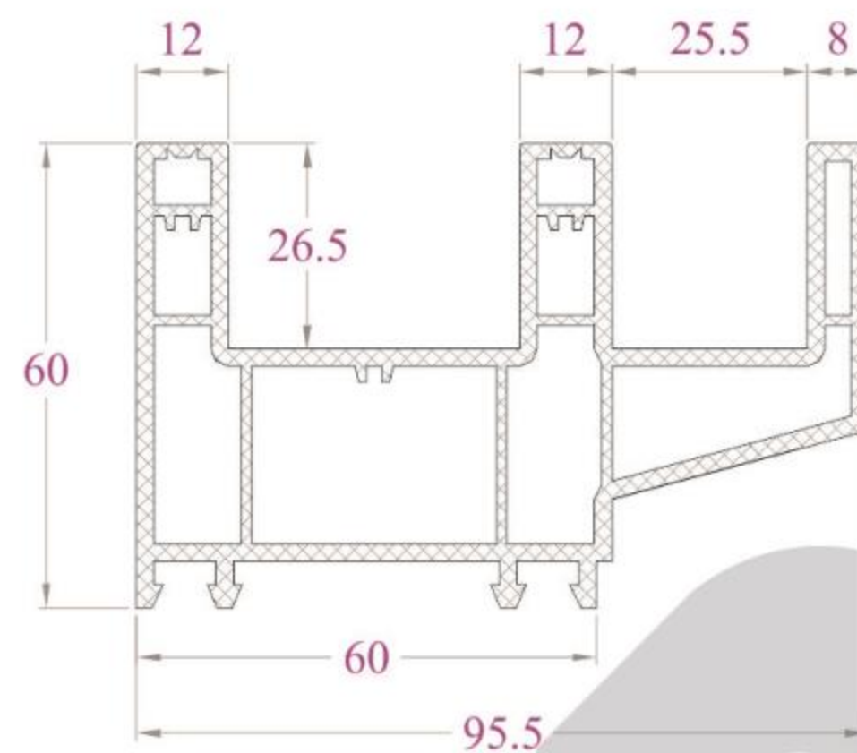
KHUNG CỬA TRƯỢT HF95NC - 1566 g/m
