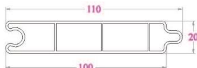
PANO CỬA - PP100N 613 g/m
