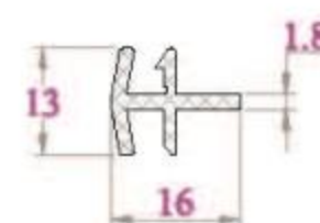
NỐI THẲNG CP2NC - 103 g/m
