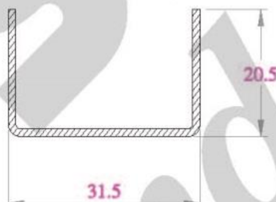
LỖI THÉP ST31.5x20.5 DÙNG CHO THANH FR73N
