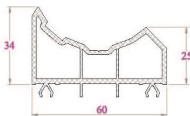
THANH GHÉP TRỤ CHUYỂN HƯỚNG ADA60NC - 663 g/m
