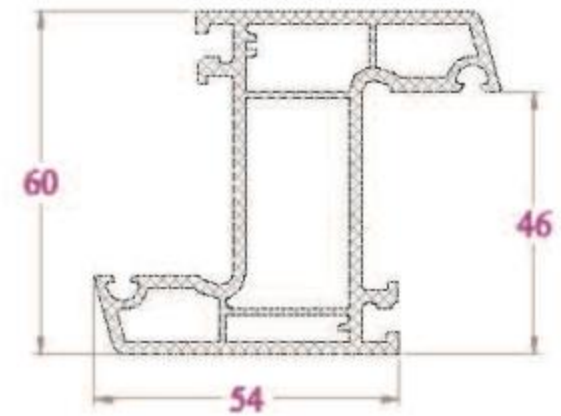
ĐỒ CỐ ĐỊNH - KP72NC 1059 g/m
