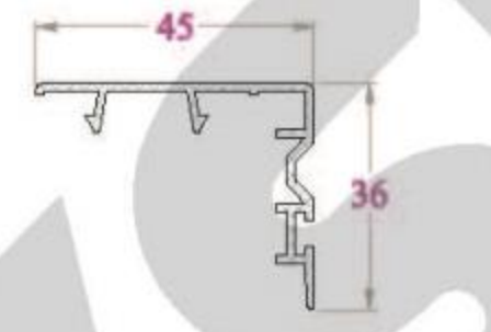
BÍT ĐẦU KHUNG - IL36NC 233 g/m
