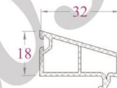
NỆP KÍNH GB31NC 272 g/m (Kính đơn 8)
