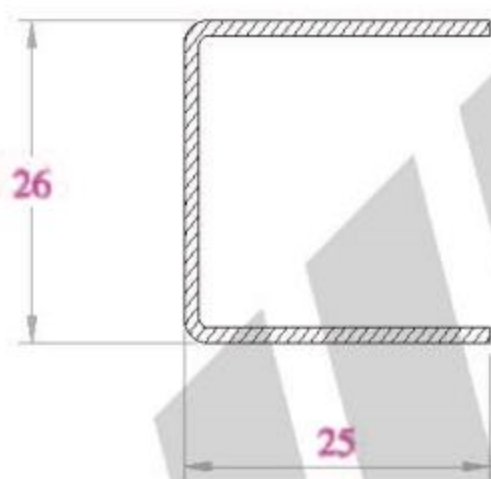
LỖI THÉP STC25x26 DÙNG CHO THANH JT61
