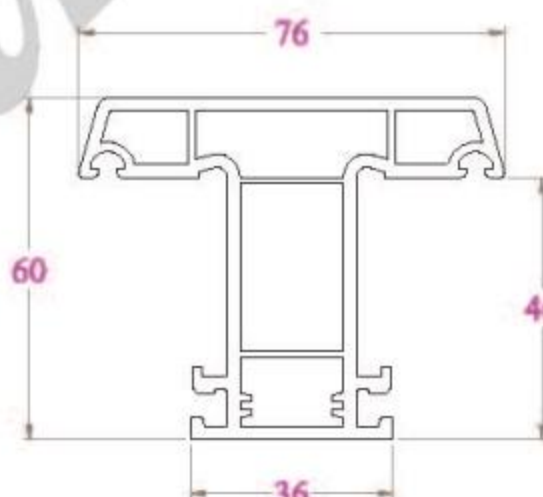
ĐỒ CỐ ĐỊNH SE76N - 1119 g/m
