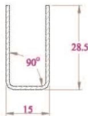
LỖ THÉP ST28.5x15 DÙNG CHO THANH SP66NC
