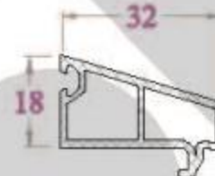
NẸP KÍNH GB31NC 272 g/m (Kính đơn 8)
