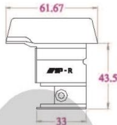
ĐẦU BÍT PHẢI DB61NC/P
