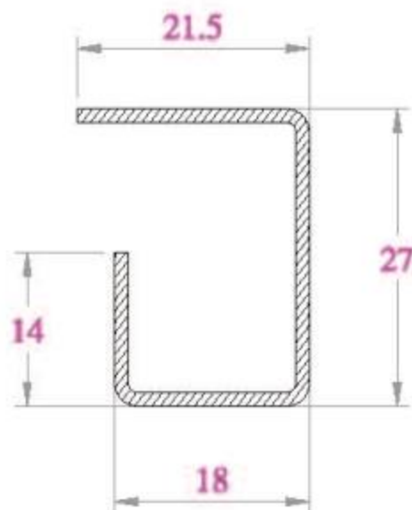
LỖI THÉP ST27x21.5 DÙNG CHO THANH BR60
