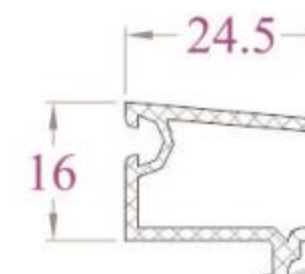
NỆP KÍNH - GB25NC 218 g/m (Kính đơn 5)
