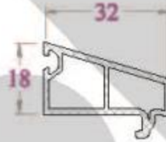
NẸP KÍNH GB31NC 272 g/m (Kính đơn 8)
