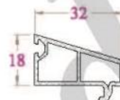
NẸP KÍNH GB31NC 272 g/m (Kính đơn 8)
