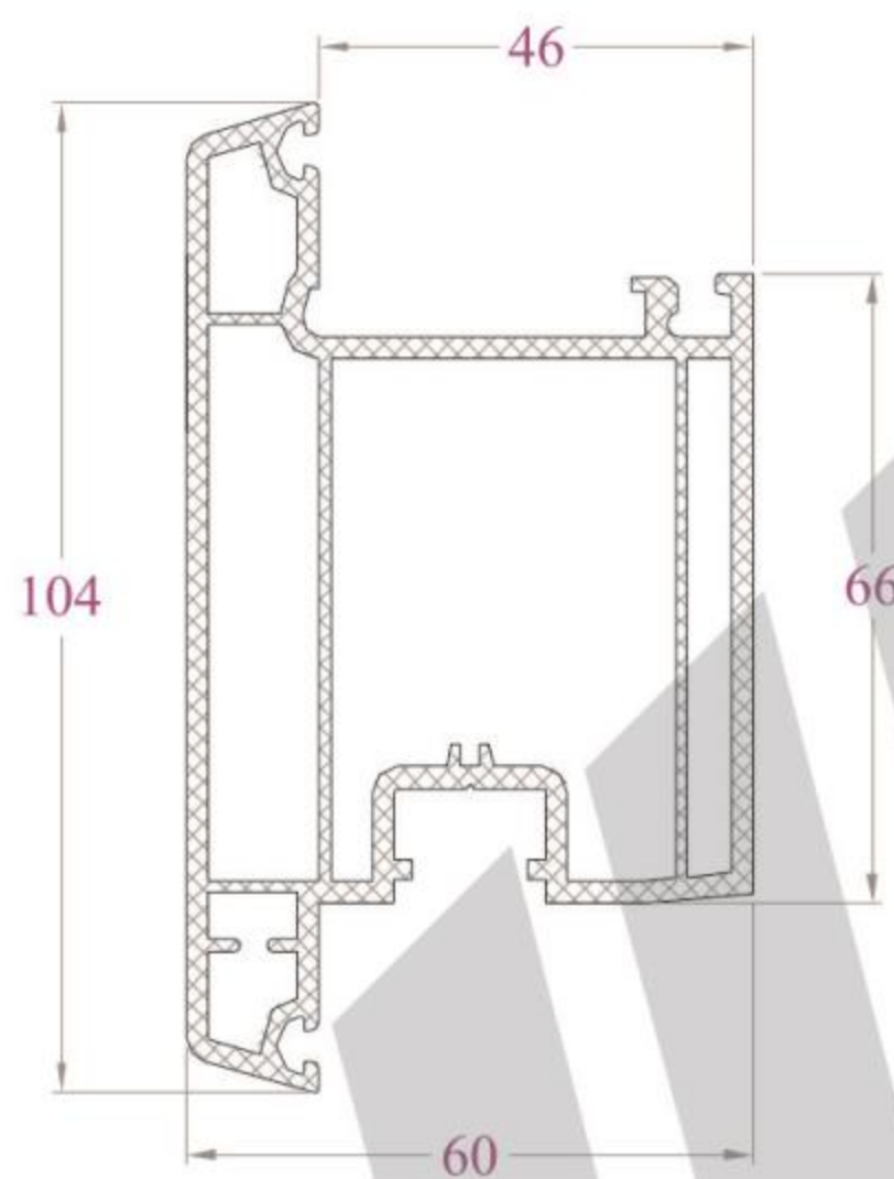
KHUÔN CỬA - SF104NC 1468 g/m
