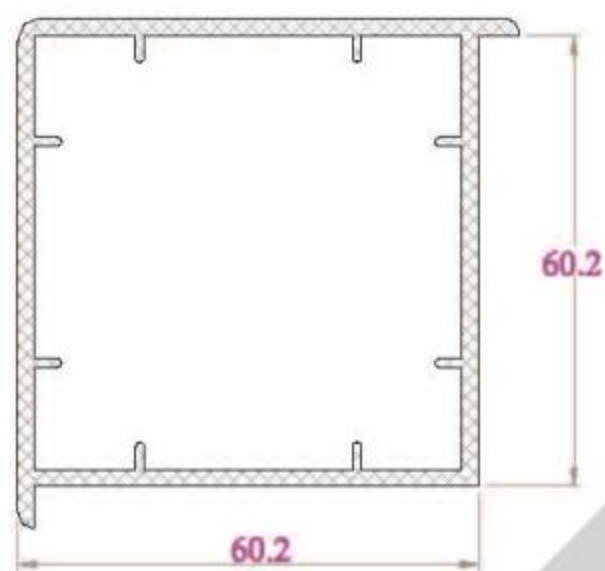
TRỤ CHUYỂN HƯỚNG 90° CP90NC - 960 g/m
