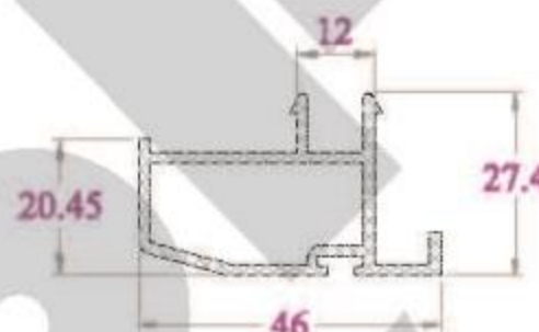
BÍT ĐÁY CỬA - HB46NC 337 g/m
