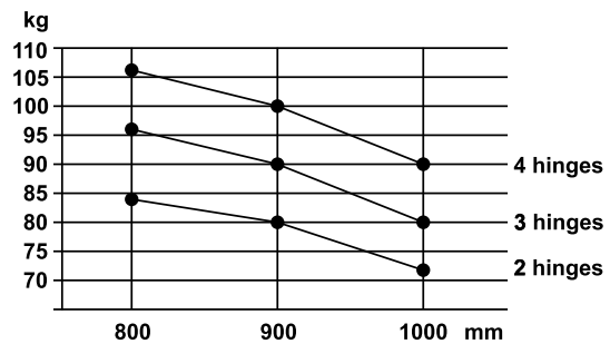
Bảng trọng lượng cửa Weight chart
