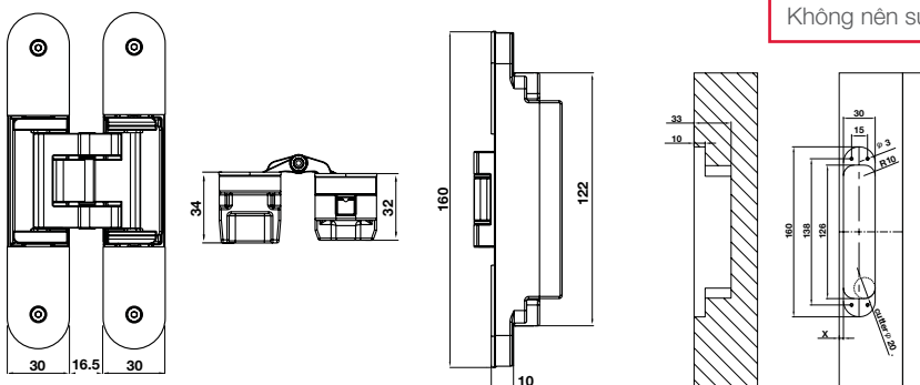
Concealed mortise hinge 3D adjustable FRH120 Bản lề âm FRH120
