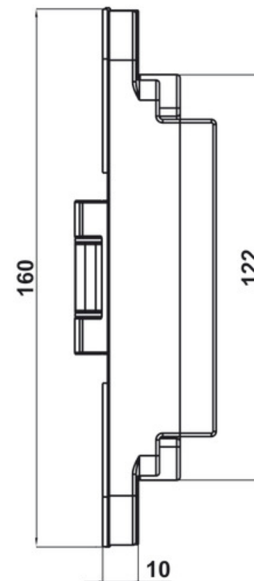
KÍCH THƯỚC MẶT BÊN
