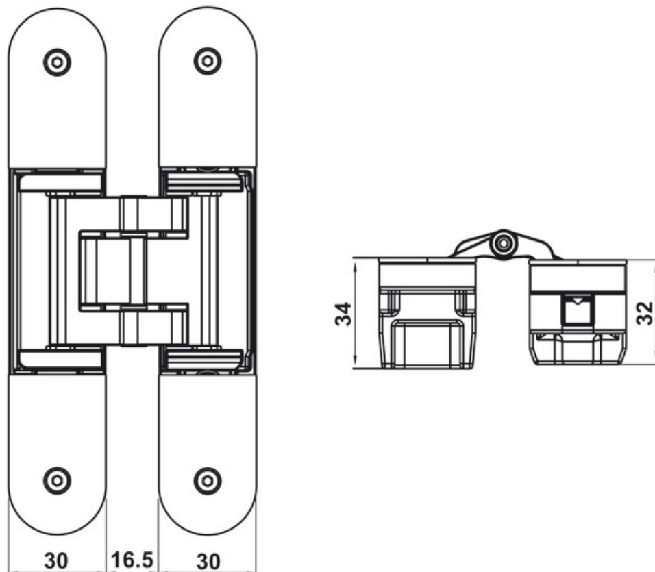
KÍCH THƯỚC MẶT TRƯỚC
