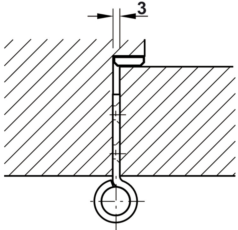
Chi tiết lắp đặt 02
