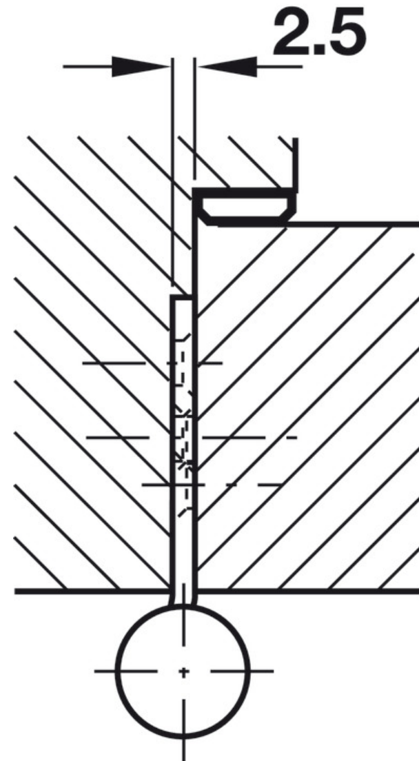
Mặt cắt lắp đặt
