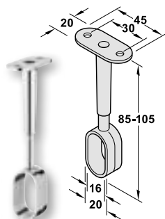
Lateral support, height adjustable Giá đỡ cạnh bên, có thể chỉnh chiều cao
