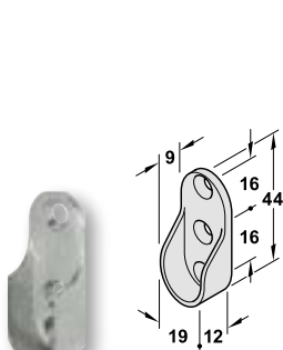
Lateral support Giá đỡ cạnh bên
