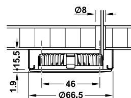
Surface mounting / Lắp nổi
