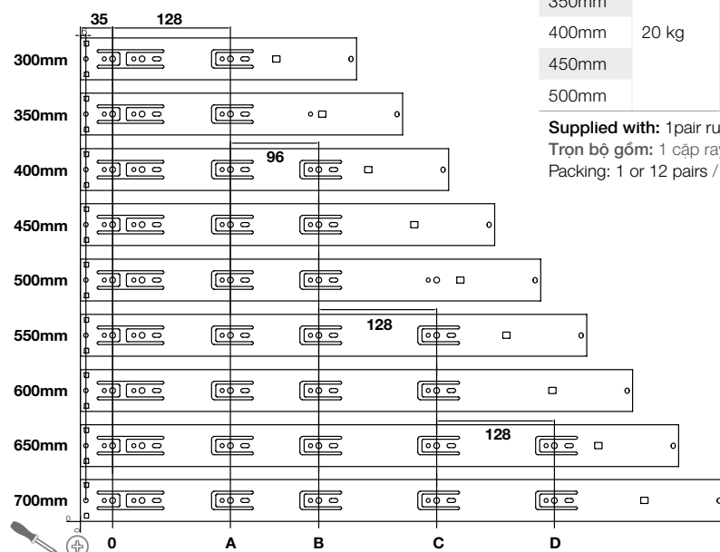
Drilling pattern / Vị trí khoan
