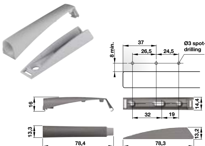
Adapter housing and plate for long version Nắp che và đế cho nêm nhấn phiên bản dài
