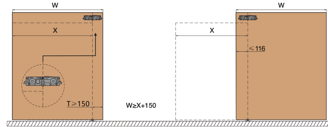
INSTALLATION 1: DOOR PARTIALLY OPEN KIỂU LẮP ĐẶT 1: CỬA MỞ KHÔNG HOÀN TOÀN
