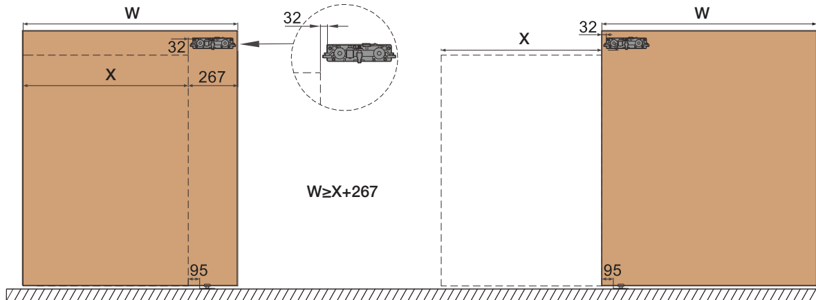
INSTALLATION 2: DOOR FULLY OPEN KIỂU LẮP ĐẶT 2: CỬA MỞ HOÀN TOÀN
